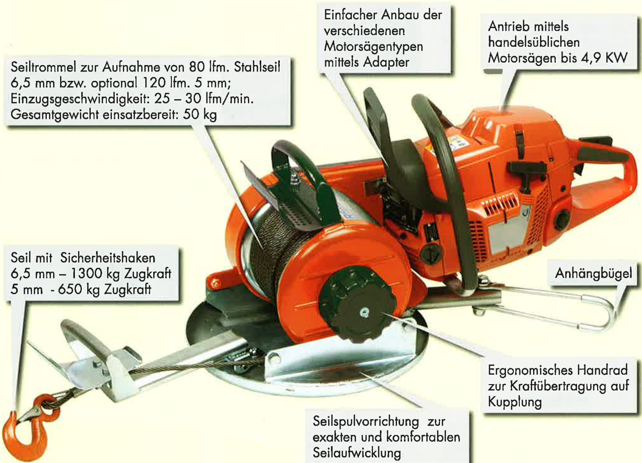
Abbildung: FKS-Compact-13 Profiplus (Sondermodell) Gesamtgewicht ohne Motorsäge: 41 kg
